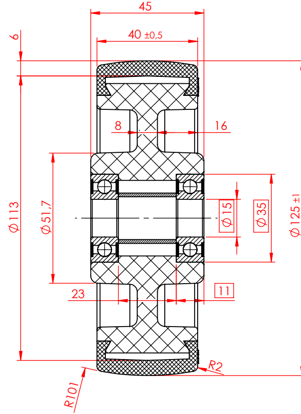
KESIT A-A ÖLÇEK 1 : 1.5
