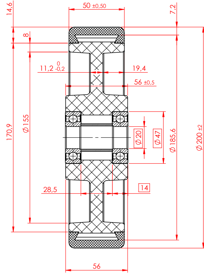
KESIT A-A ÖLÇEK 1 : 2
